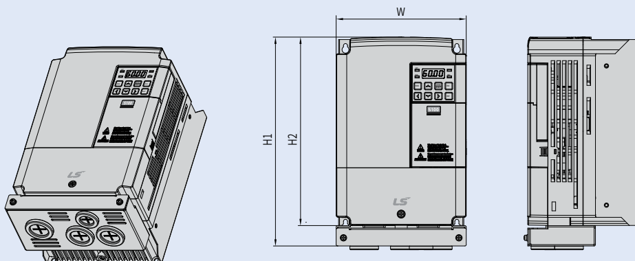
Drive + Conduit
